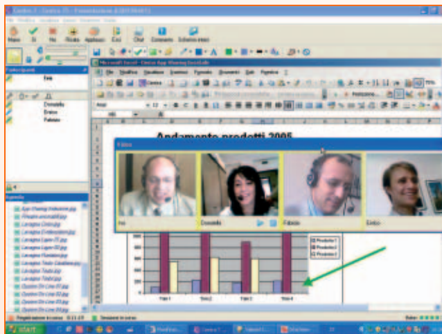
Interfaccia utente e gestione multivideo
